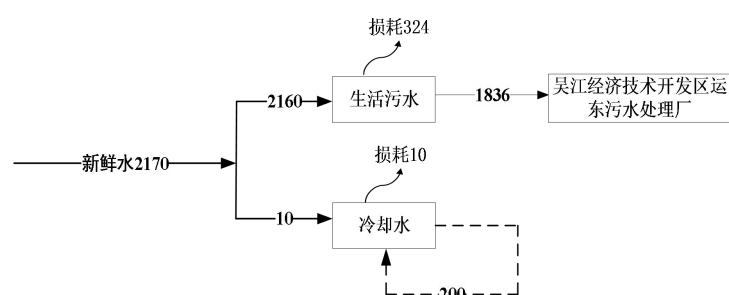
图 5-6 本项目水平衡图 单位：t/a
