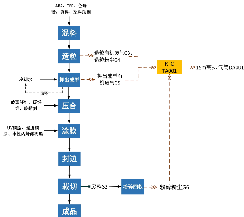
图 5-4 本项目塑料制品生产工艺流程图
