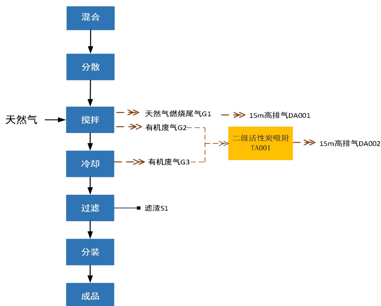
图 1-1 现有项目生产工艺流程图
