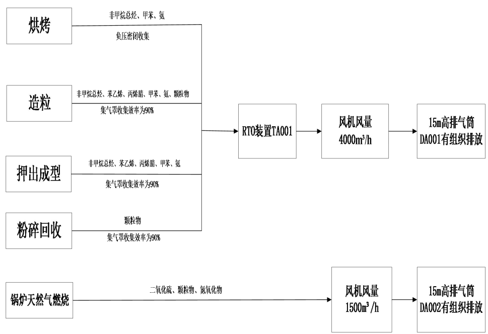
7-1 本项目废气收集、处理、排放流程示意图
