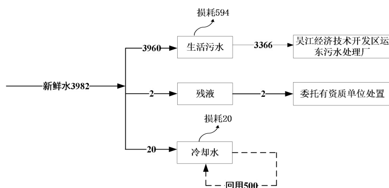
图 5-7 全厂水平衡图 单位：t/a
