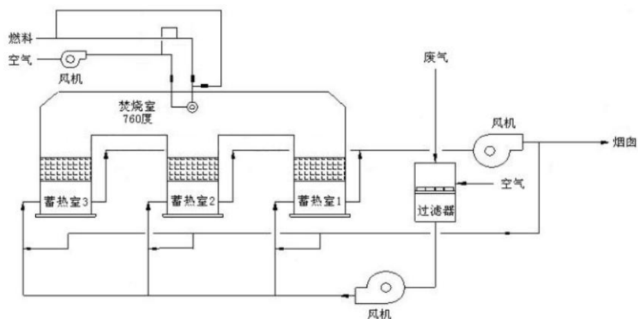
图7-3 蓄热氧化（RTO）原理图
