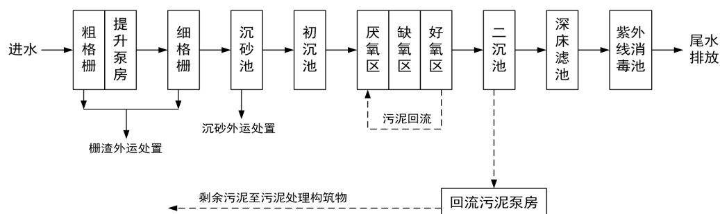
图 7-4 吴江经济技术开发区运东污水处理厂处理工艺流程图
