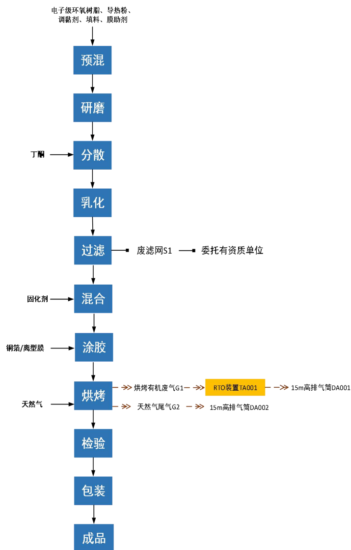
图 5-1 本项目高导热涂胶铜箔及胶膜生产工艺流程图
