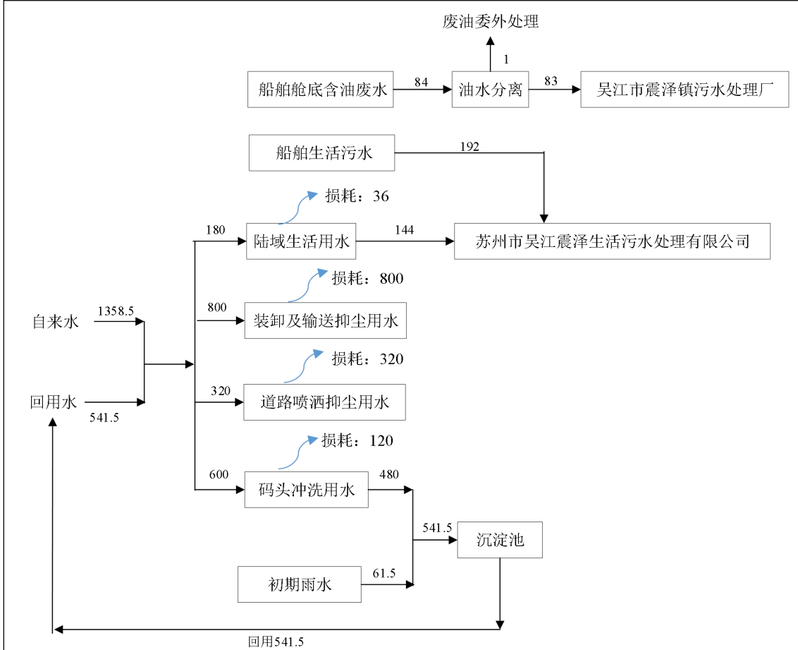
图 5-2 项目水平衡图
