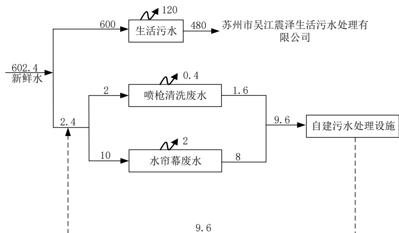
图 2-2 项目水平衡图 单位：t/a
