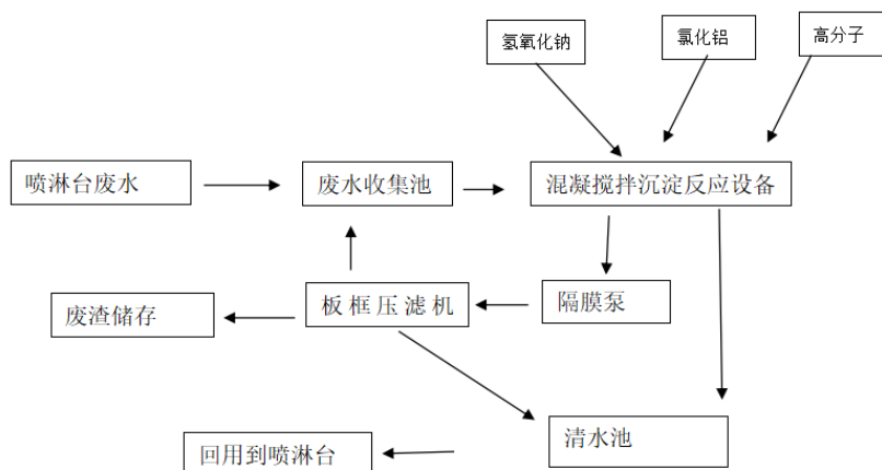
图4-2 自建污水处理设施处理工艺流程图
