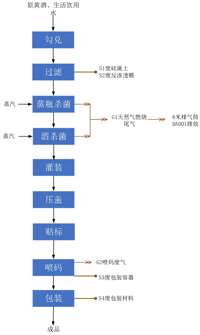
图 2-3 生产工艺及产污环节图
