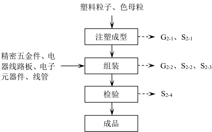
图 2-2 本项目新能源汽车配件生产工艺流程图
