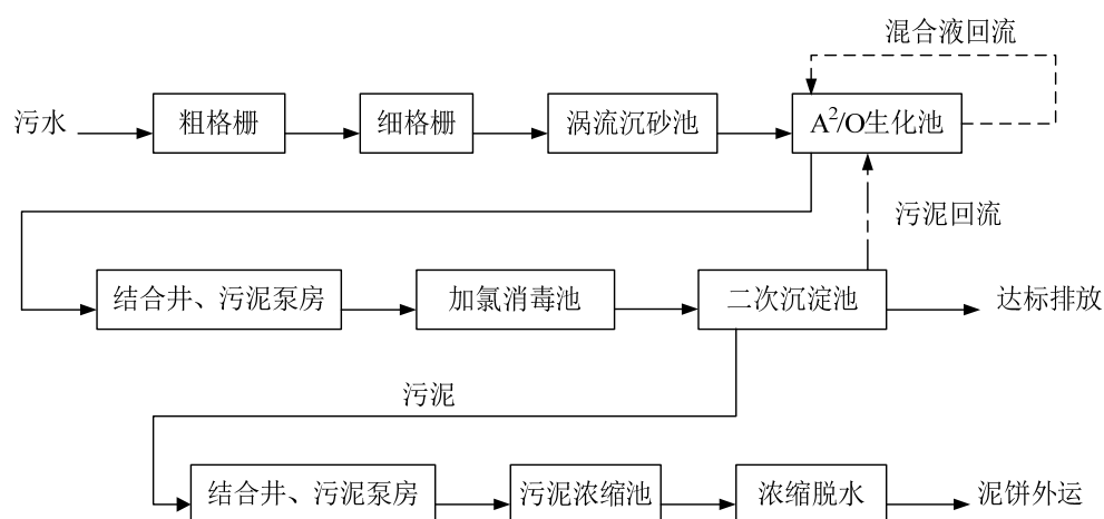
图 4-3 污水处理厂工艺流程
