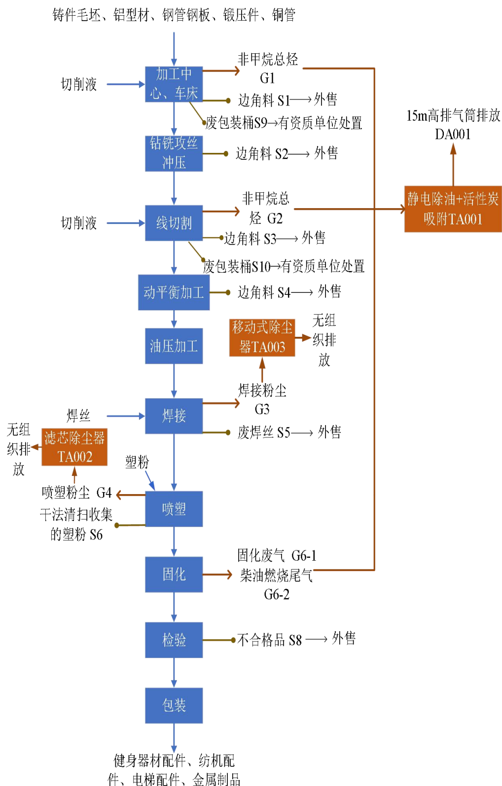
图 3-6 生产工艺流程图
