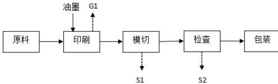
图 2-2 不干胶标贴生产工艺流程图
