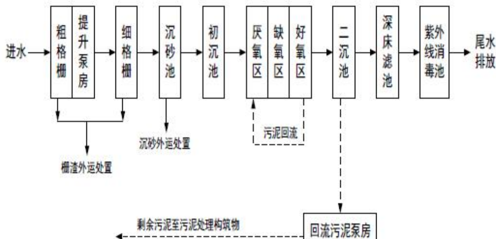
图 4-3 吴江经济技术开发区运东污水处理厂处理工艺流程图
