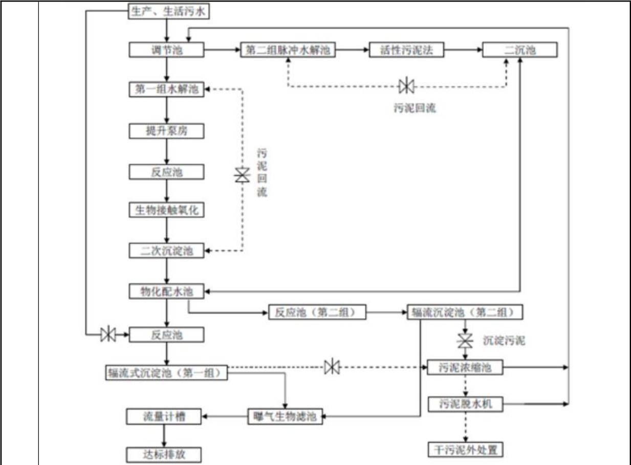
图 4-2 污水处理工艺流程图
