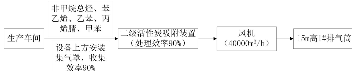
图 4-1 本项目废气收集走向示意图
