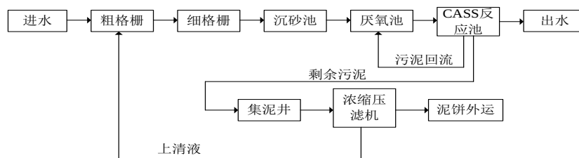
图 4-3 苏州市吴江经济技术开发区运东污水处理有限公司工艺流程图
