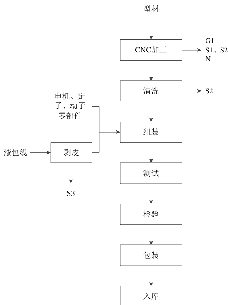
图 2-1 生产工艺流程图
