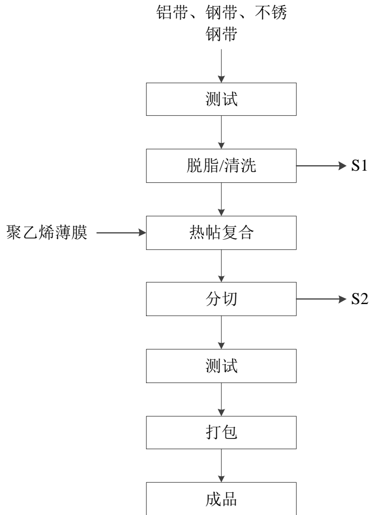
图 2-1 生产工艺流程图
