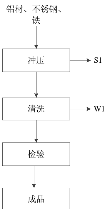
图 2-1 精密五金件生产工艺流程图
