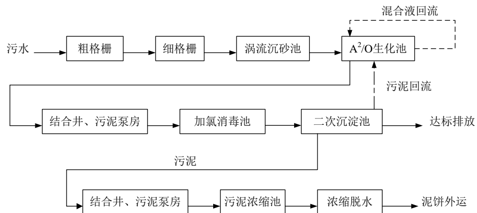
图 4-3 苏州市吴江城南污水处理有限公司污水处理工艺流程图
