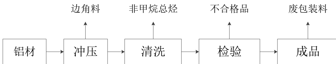
图 2-1 高档五金件生产工艺流程图
