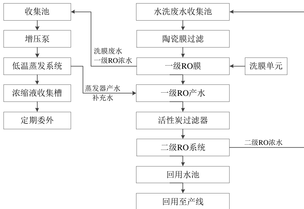
图 4-2 本项目污水处理系统设备工艺流程图
