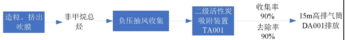
图 4-1 废气处理流程图
