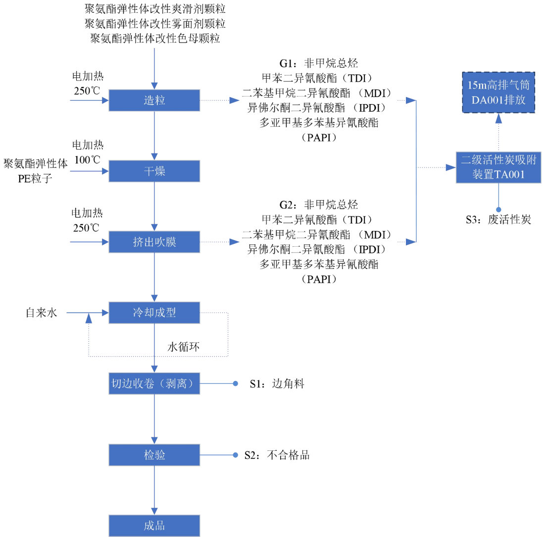
图 2-2 生产工艺流程图
