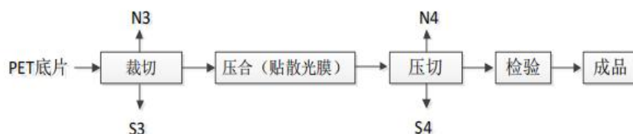
图 1-2 扩散片工艺流程图
