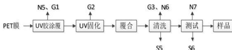
图 1-3 光学材料工艺流程图
