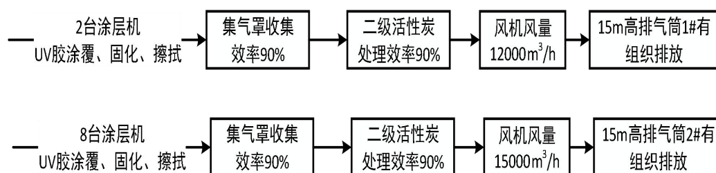
图 4-1 本项目废气处理流程图
