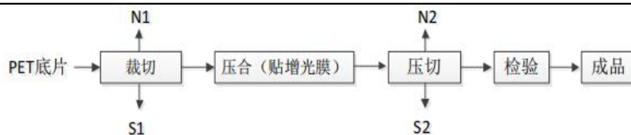
图 1-1 增光片工艺流程图
