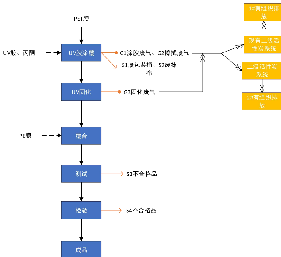
图 2-2 电子元器件产线工艺流程图
