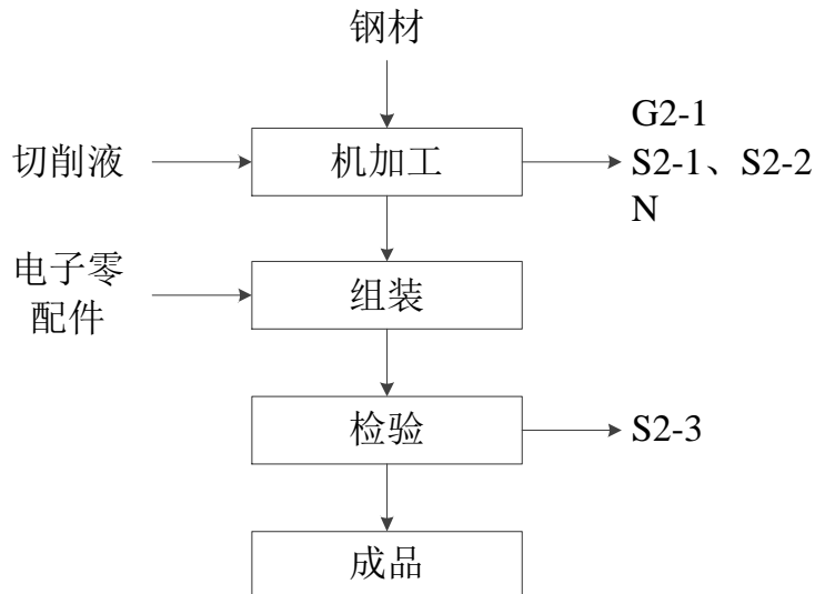
图 2-3 自动化设备生产工艺流程图
