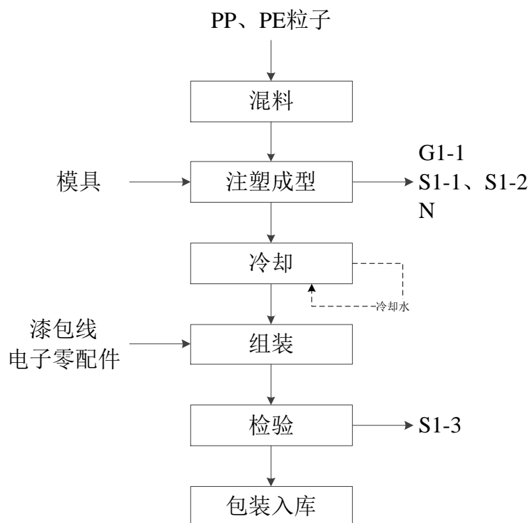
图 2-2 汽车连接器生产工艺流程图
