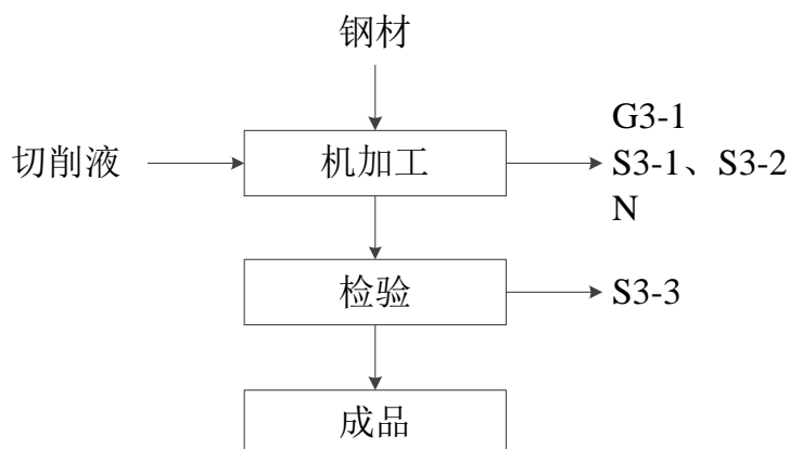
图 2-4 精密模具生产工艺流程图
