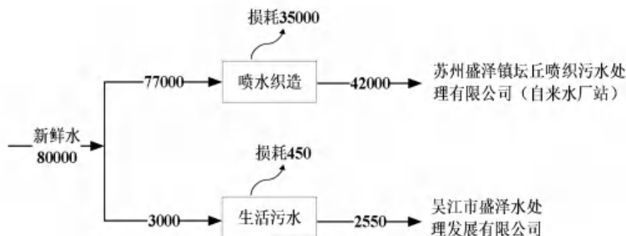
图 2-5 吴江市林超纺织厂水平衡图 (t/a)
