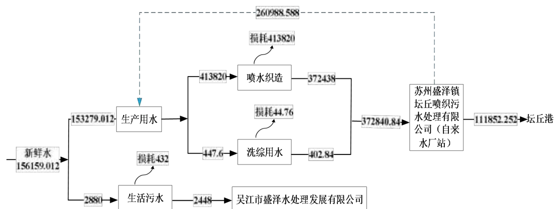
图 2-1 改建后全厂水平衡图 (t/a)
