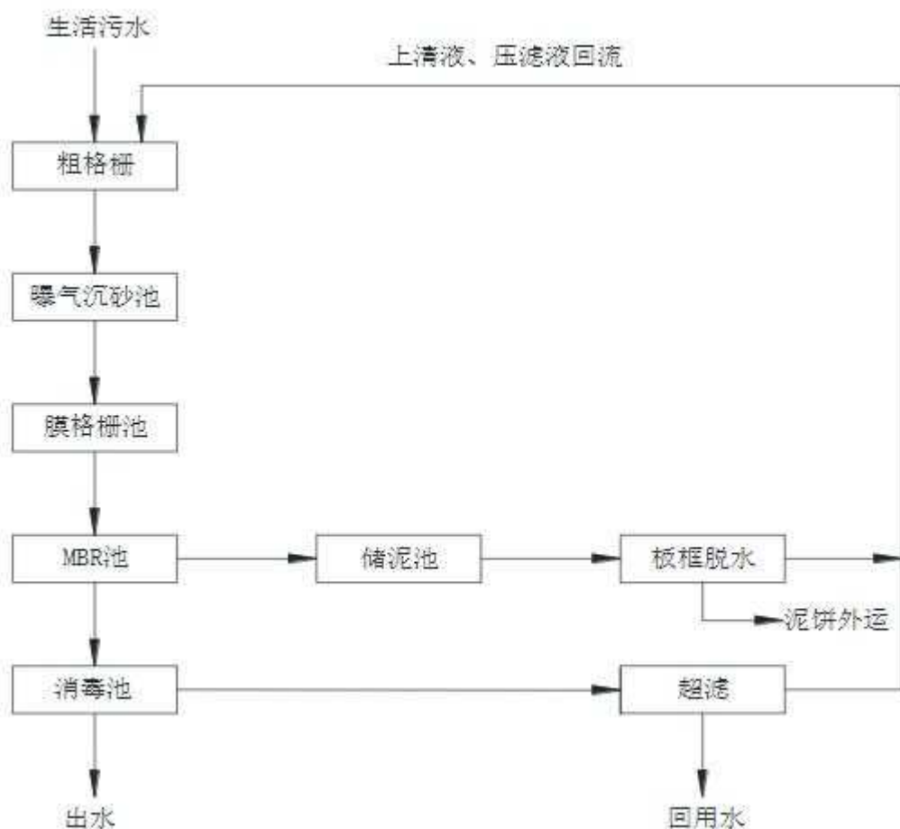
图 4-1 吴江市盛泽水处理发展有限公司工艺流程图
