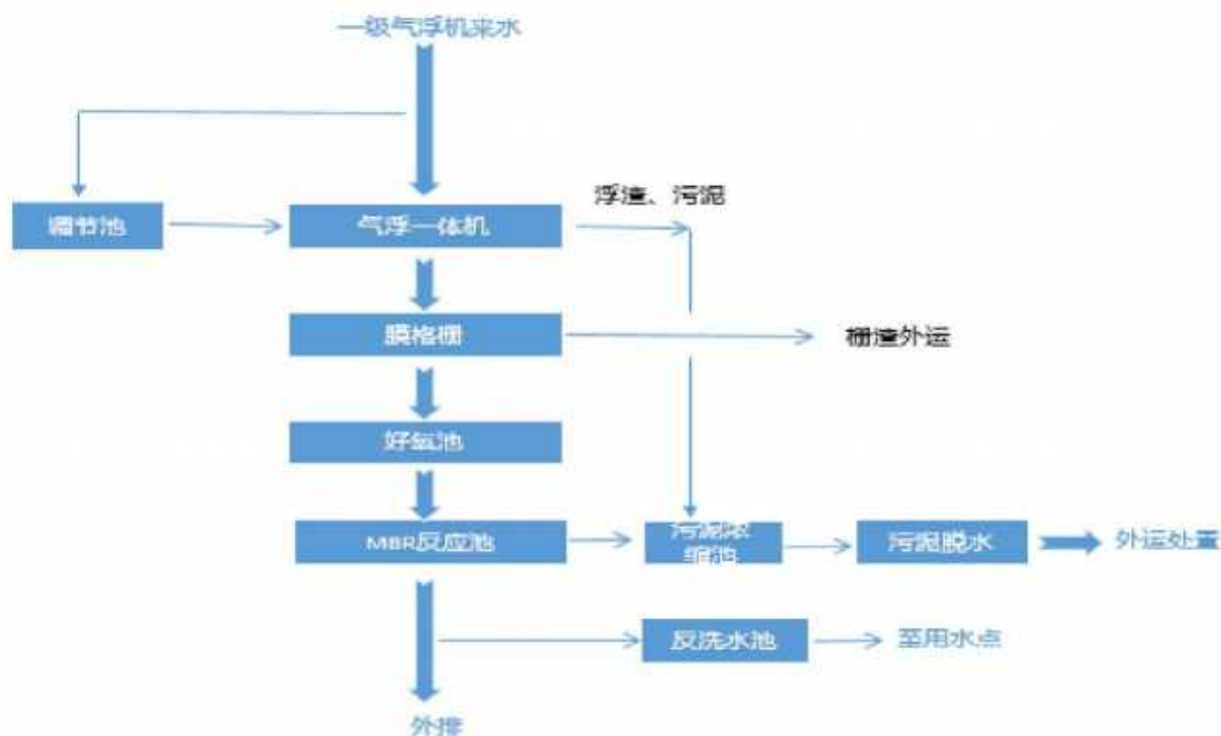
图 4-2 苏州盛泽镇坛丘喷织污水处理有限公司（自来水厂站）工艺流程图 A、废水量的可行性分析
