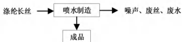
图 2-4 喷水织造生产工艺流程图
