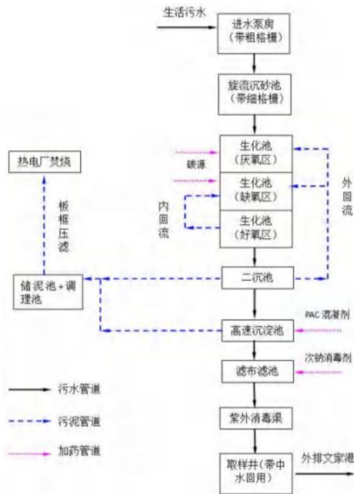
图 4-1 苏州市吴江桃源生活污水处理有限公司工艺流程图 A、废水量的可行性分析
