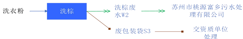
图 2-3 洗棕生产工艺流程图
