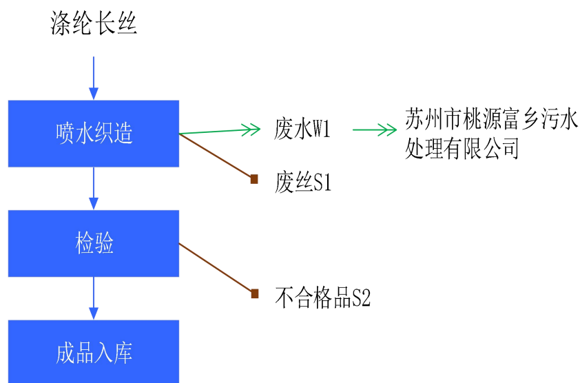
图 2-2 喷水织造生产工艺流程图
