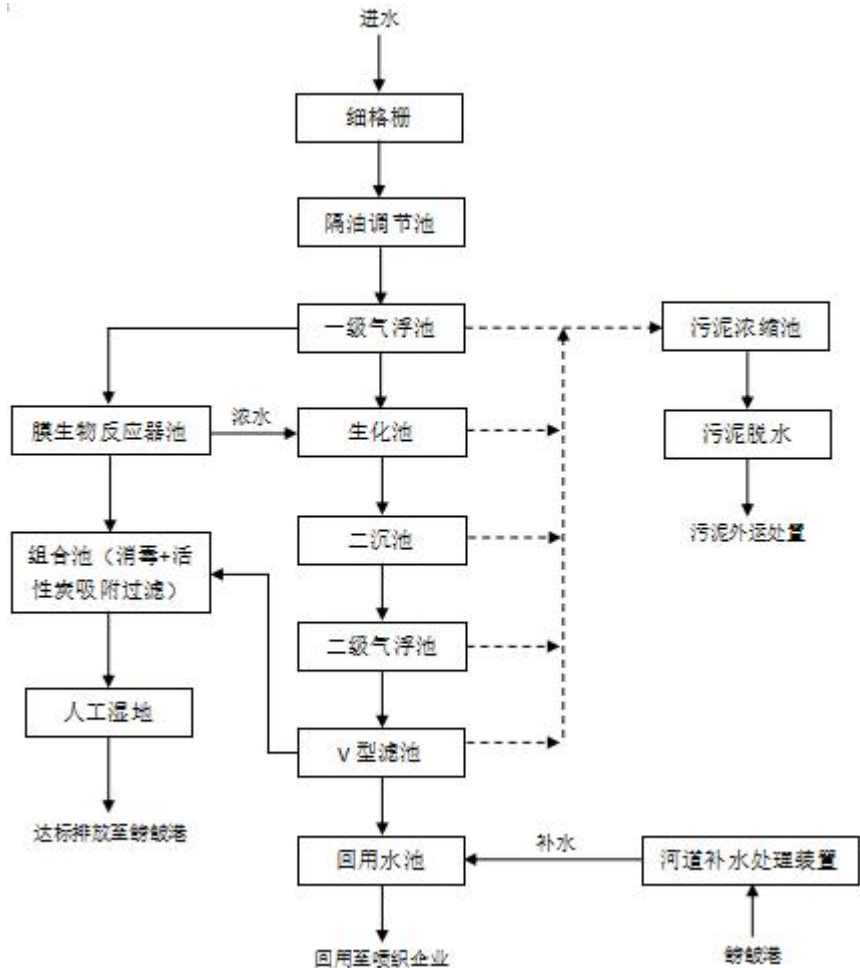
图 4-2 苏州市桃源富乡污水处理有限公司废水处理工艺流程图
