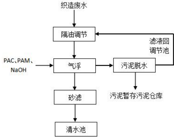
图 4-1 现有污水处理设施废水处理工艺流程图
