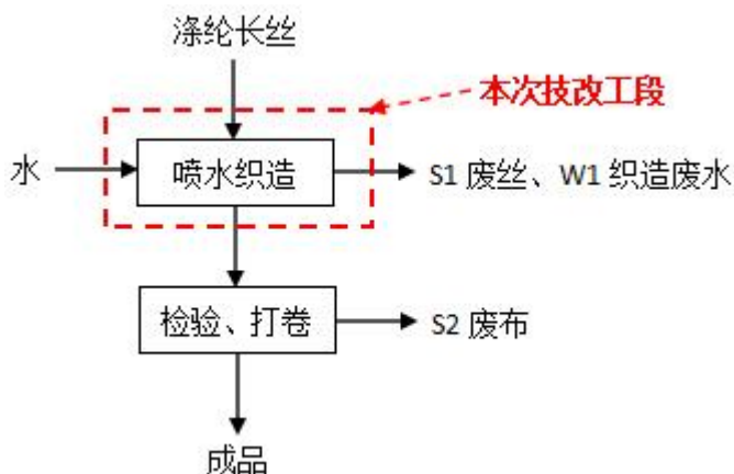
图 2-3 本次搬迁（改造）项目生产工艺流程及产污环节示意图
