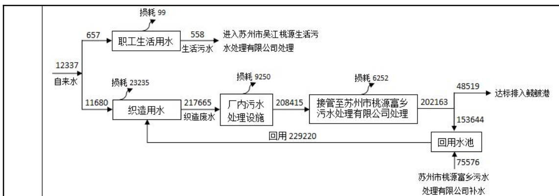
图 2-1 项目搬迁后水平衡图 (单位: t/a)
