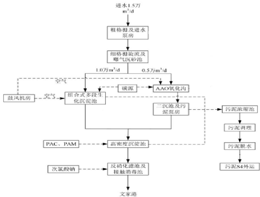
图 4-3 苏州市吴江桃源生活污水处理有限公司废水处理工艺流程图
