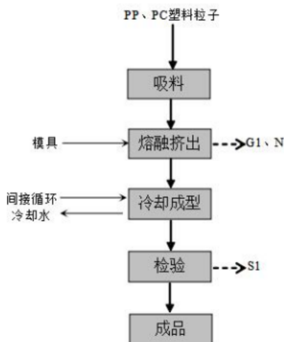
图 2-2 生产工艺流程图
