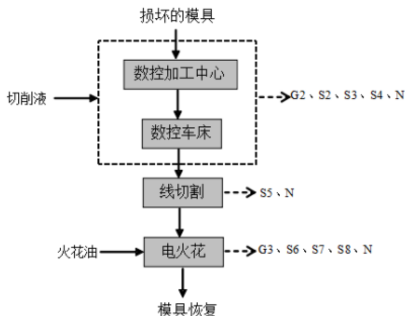
图 2-3 模具维修工艺流程图
