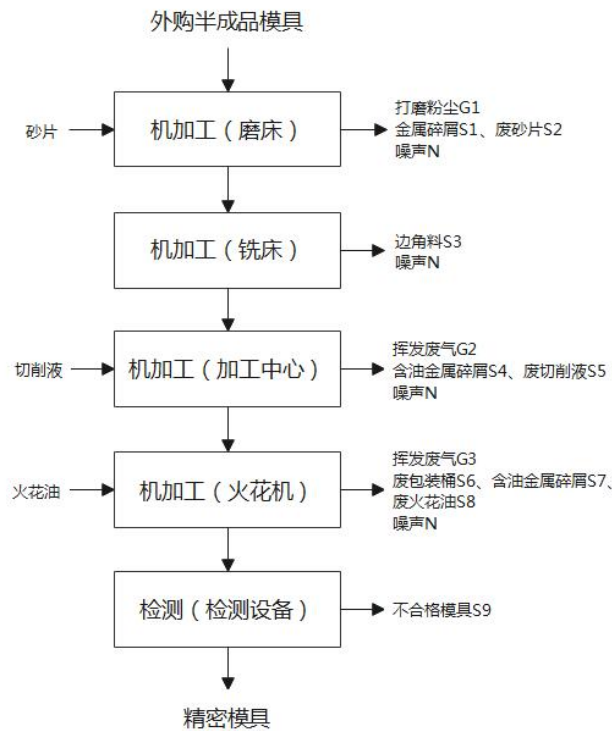
图 2-2 本项目模具生产工艺流程图
