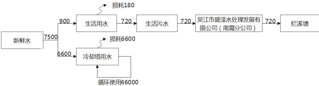
图 2-1 本项目水平衡图 (t/d)
