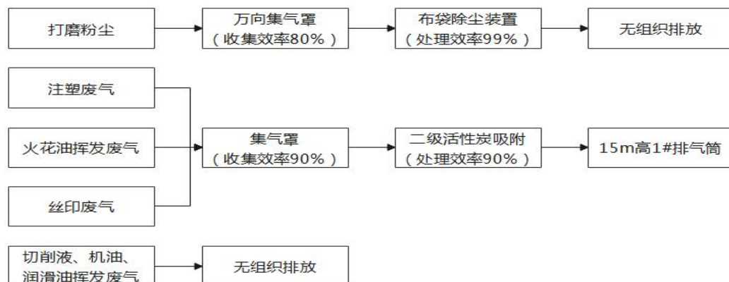
图 4-1 废气收集处理走向示意图
