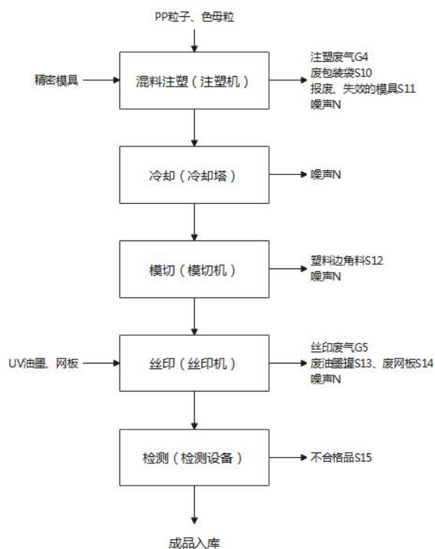
图 2-3 本项目注塑件生产工艺流程图
