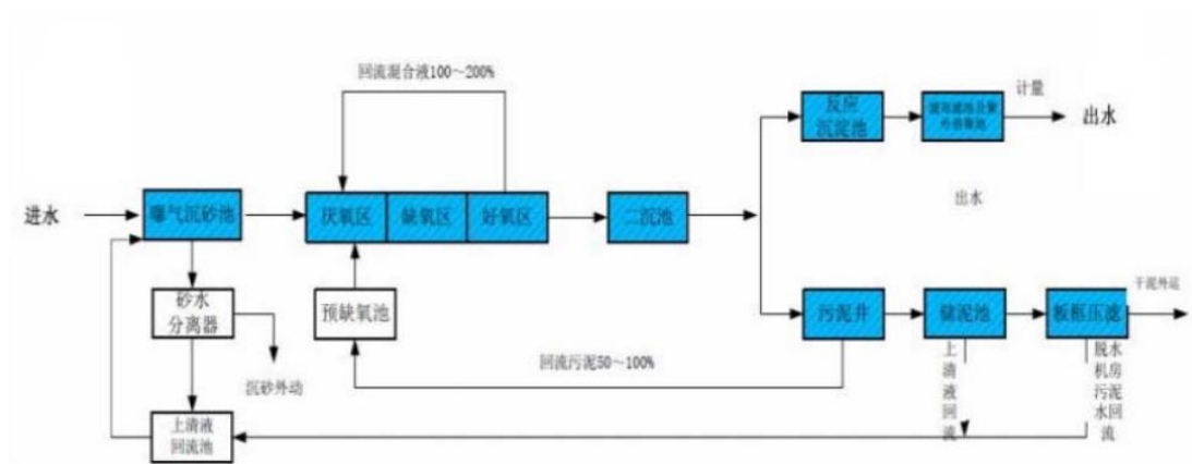
图 4-3 吴江市盛泽水处理发展有限公司（南霄分公司）二期生活污水处理工艺流程图
