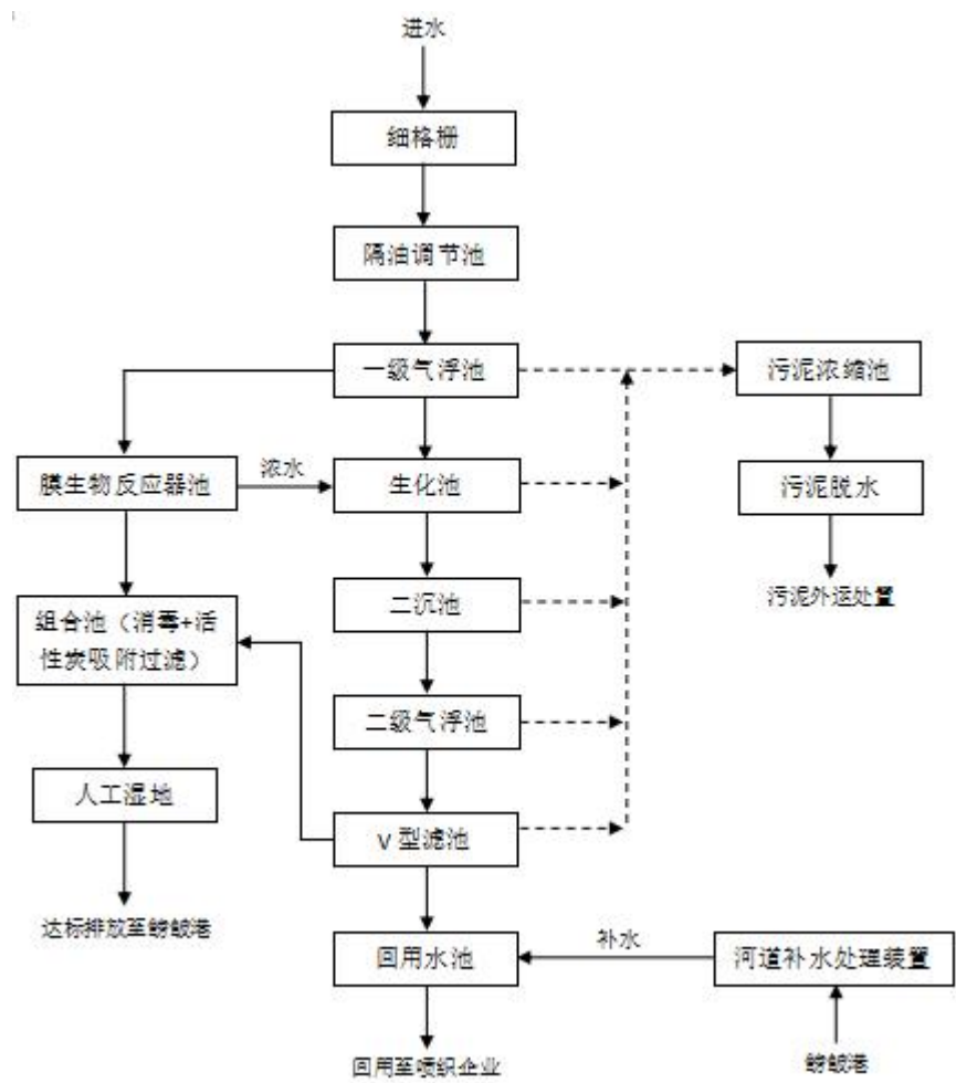
图 4-1 苏州市桃源富乡污水处理有限公司废水处理工艺流程图
