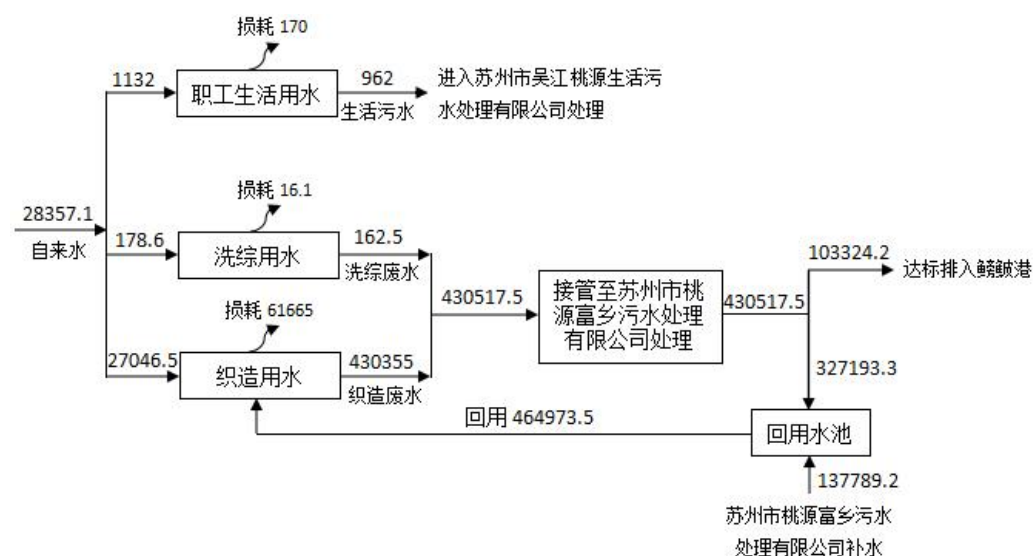
图 2-1 本项目技改后全厂水平衡图（单位：t/a）
