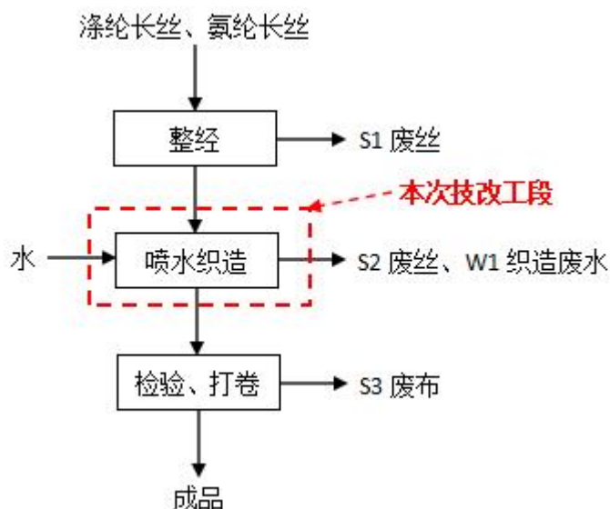
图 2-3 本次技改项目生产工艺流程及产污环节示意图
