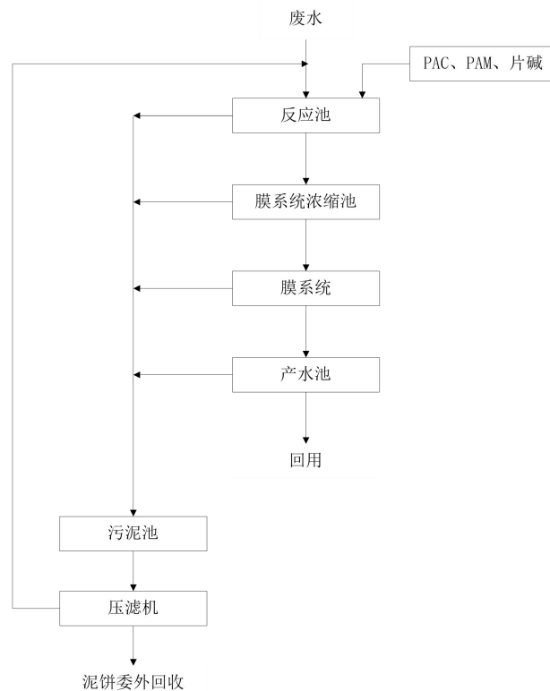
图 4-2 本项目污水处理工艺流程图
