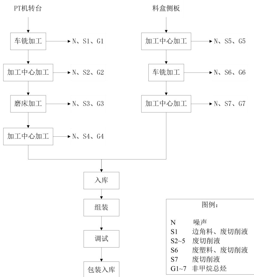
图 2-4 年产双头双轨、单头单轨太阳能电池丝网印刷线工艺流程图 工艺说明：
