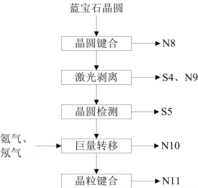
图 2-5 巨量转移设备测试工艺流程图
