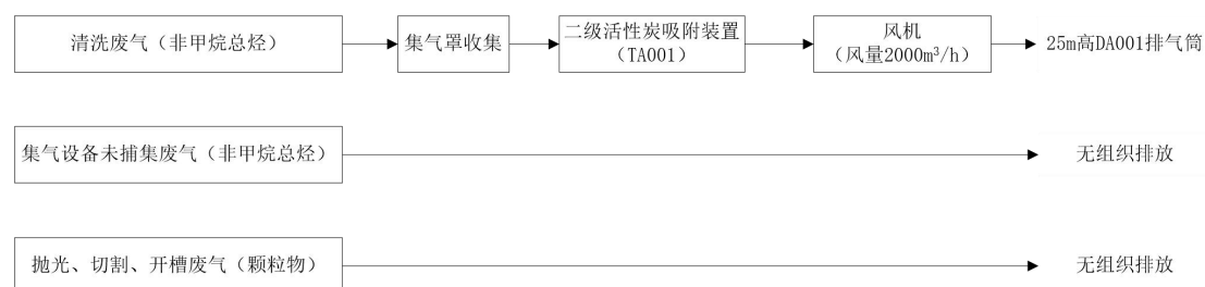
图 4-1 本项目废气收集图
