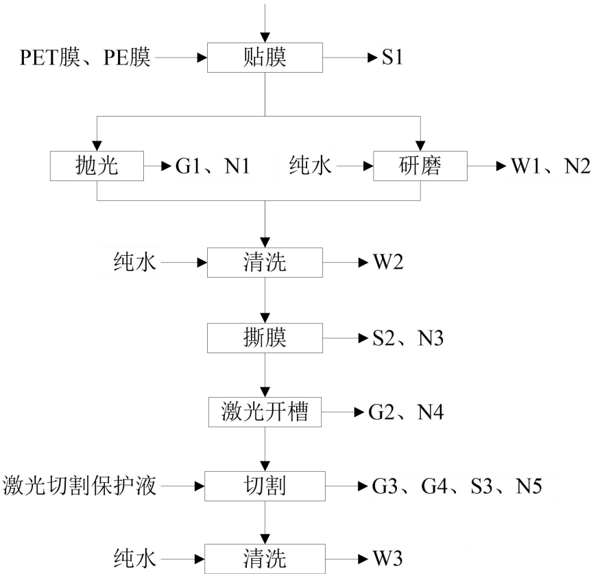
图 2-3 磨划设备测试工艺流程图
