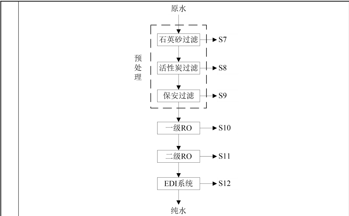
图 2-7 纯水制备工艺流程图
